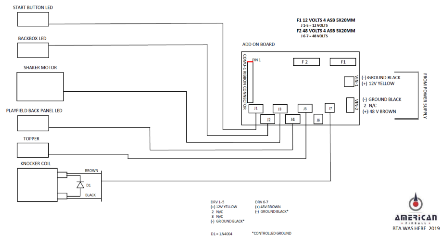
ADD ON BOARD WIRING OKTOBERFEST
